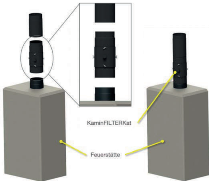
Abbildung 3: Einbaubeispiel an einer schematischen Feuerstätte
